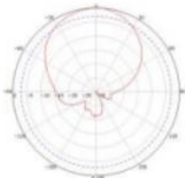
H-Plane
