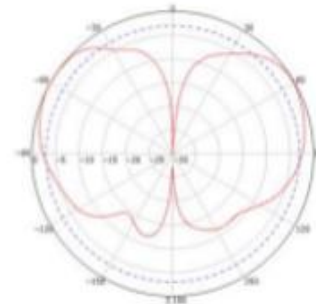
V-Plane
